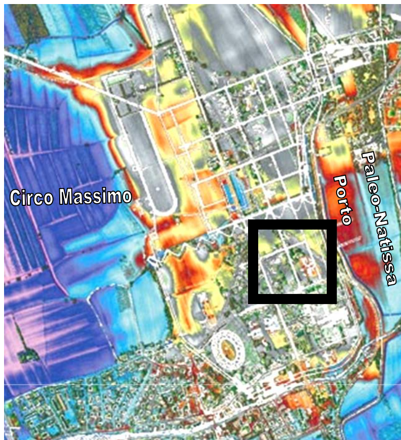
Modello digitale del terreno a conturaggio colorimetrico sulla scala delle altezze. Con i colori chiari sono evidenziate le aree a quota più elevata. E' evidenziato il sito in esame ed il paleo-alveo del T.Natissa (Rilievo estratto da Coren, Visintini, Fales, Sterzai, Prearo, Rubinich, 2005).
