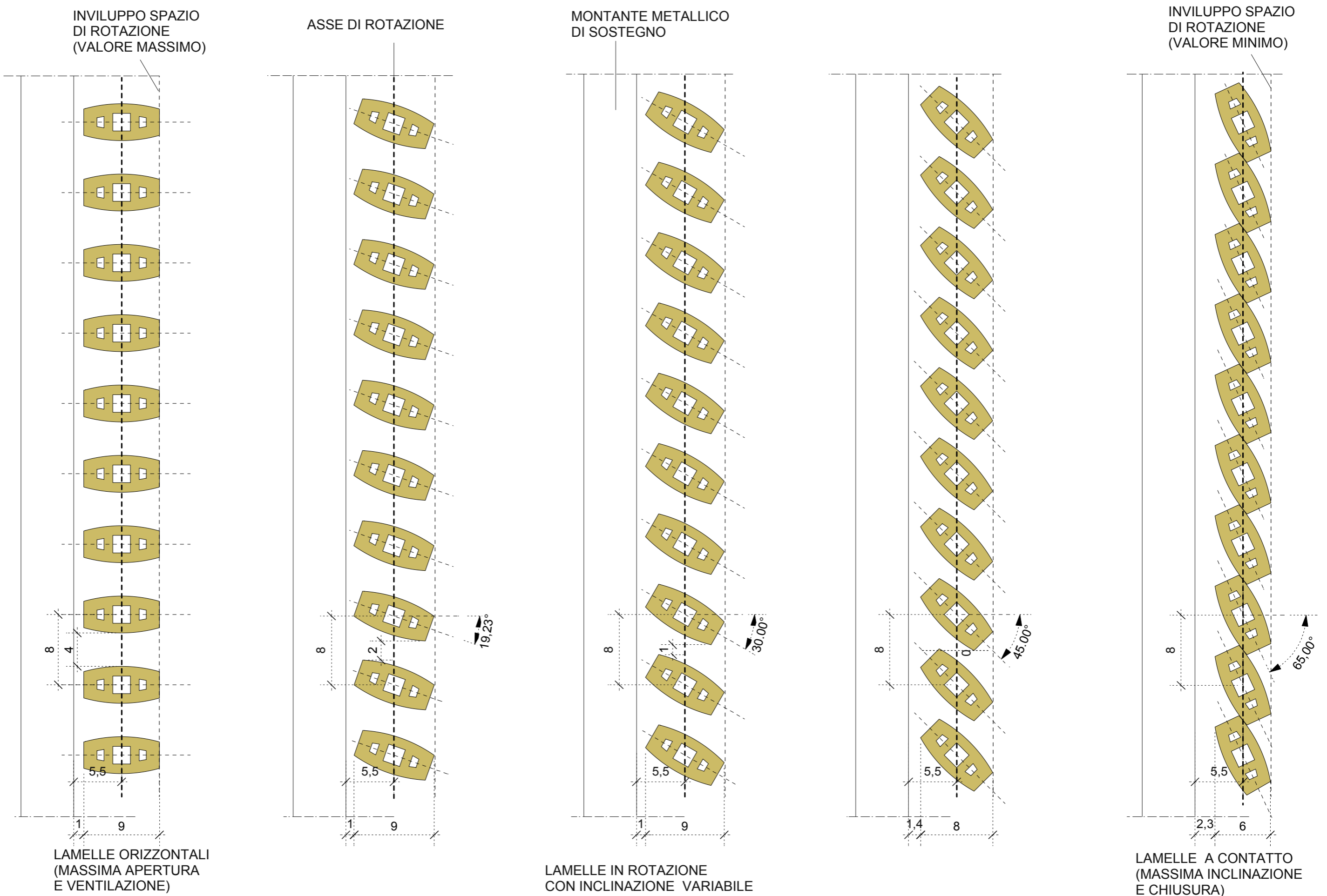
PIANTA-TIPO 1: 20
