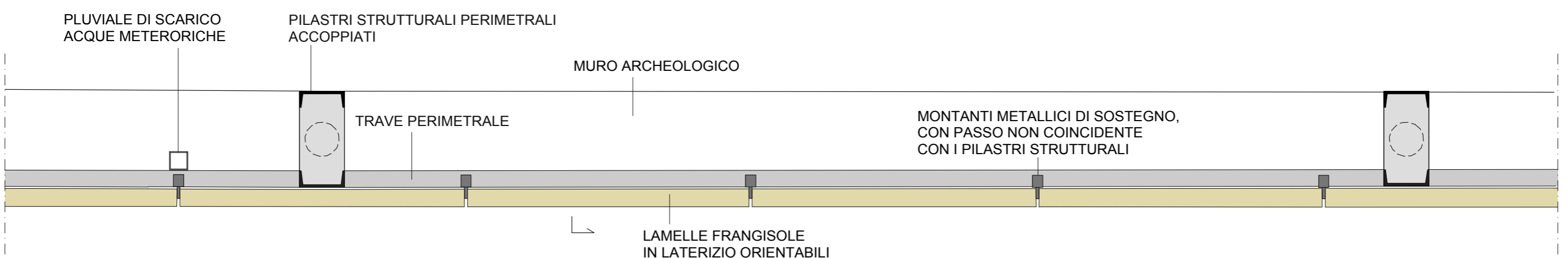
PIANTA-TIPO 1: 20
